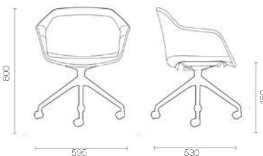
Toumant 4 branches polyamide noir ou blanc sur roulettes Ø 50 sol textile. Rotating 4 arm polyamide black or white on casters Ø 50 textile floor.
